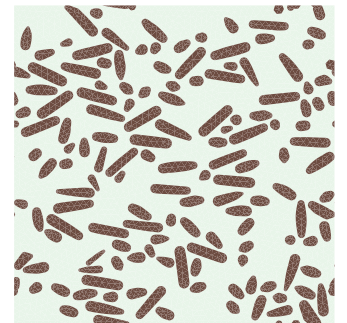
filler=0.3
